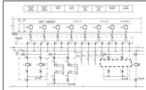
Câblage électrique du bobinage
